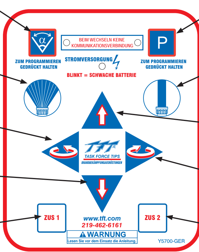
Abb. 2.2.5 Aufkleber Bedienung
