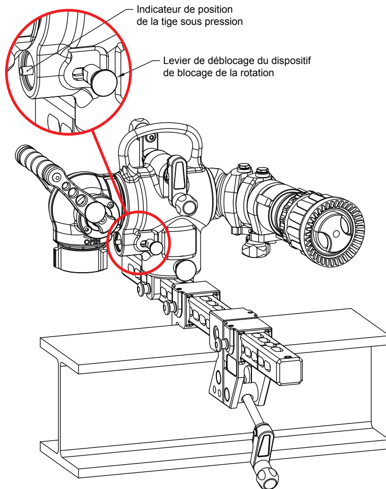
La Figure 2.34 Monitor monté sur l'ossature montrant la position du levier de déblocage du dispositif de blocage et la tige indicatrice.
