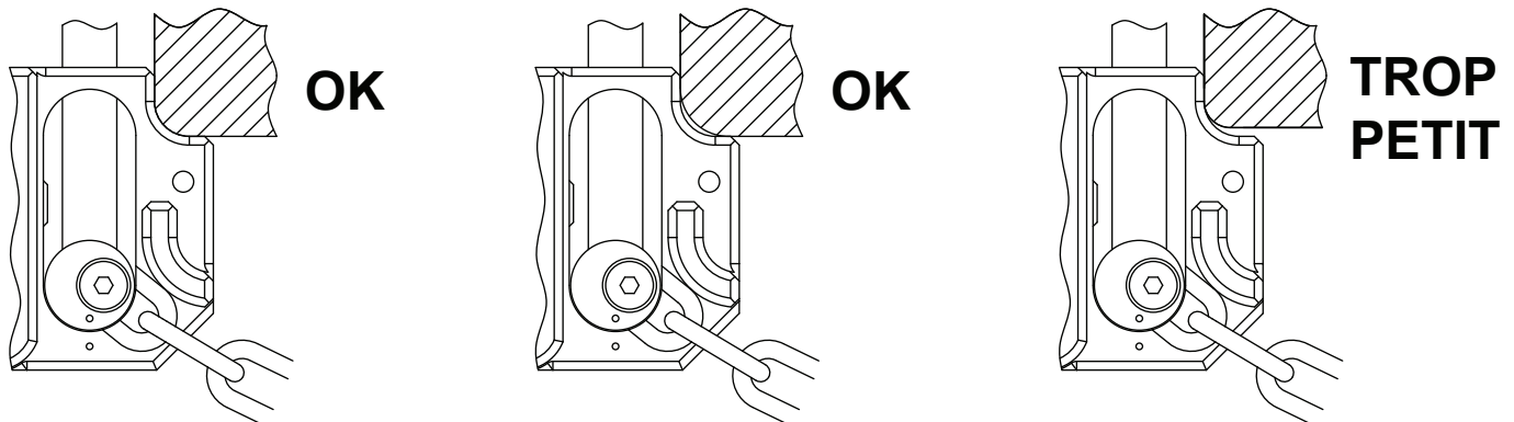
La Figure 2.19 Lecture du calibre de rayons de coins
