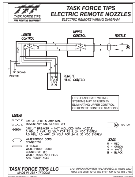
LIM-040 ER Nozzle Wiring Diagram
