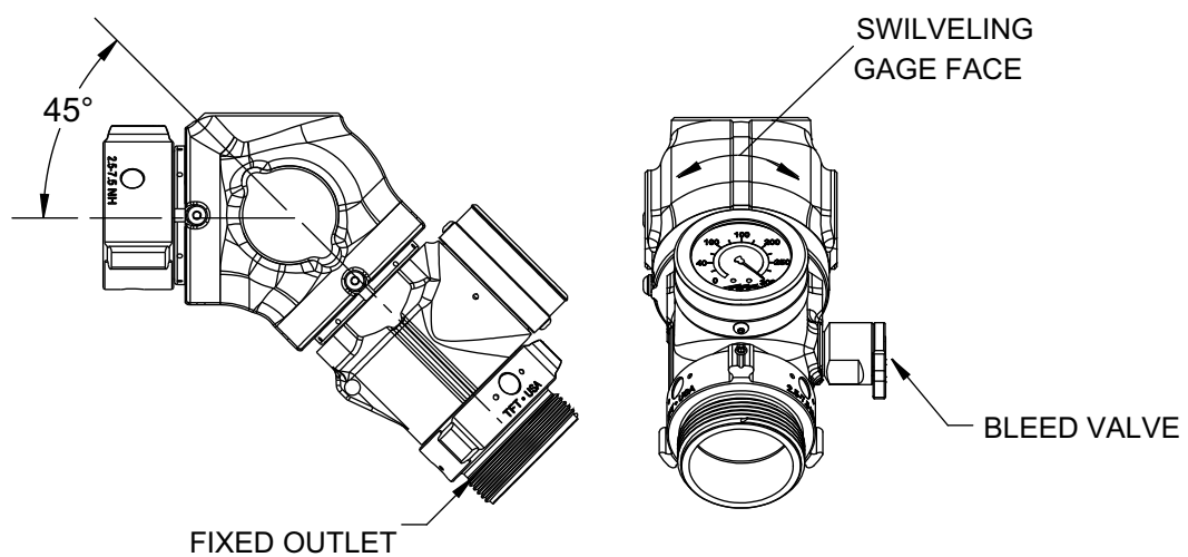
2.5" IN-LINE 45°
