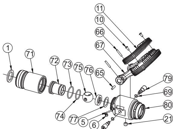
C - GD907 SUBASSEMBLY
