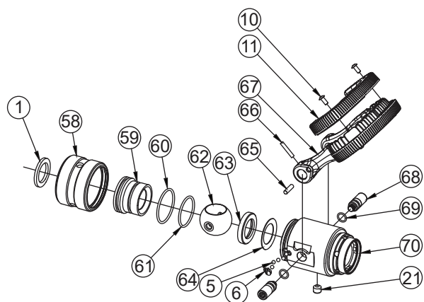
B - GD906 SUBASSEMBLY
