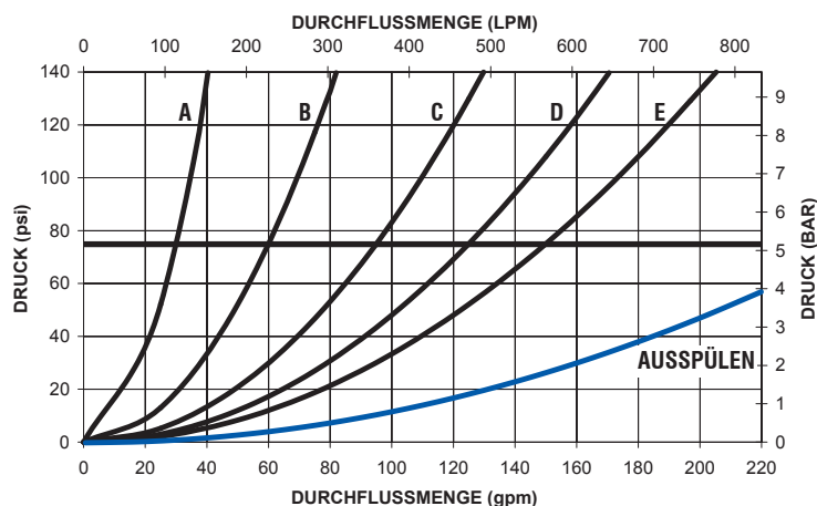
Abb. 4.2 Durchfluss-Grafik für die fest eingestellte und die variabel einstellbare Hohlstrahlrohre G-Force
