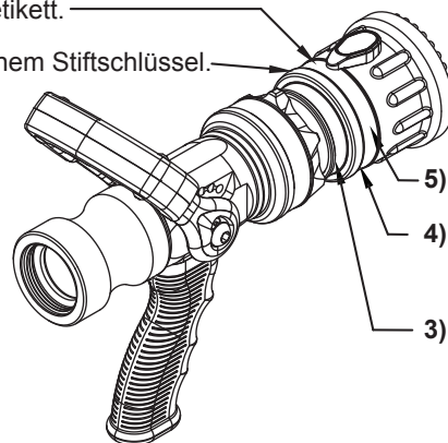
Abb. 5.2.4 Strahlmustereinstellung
